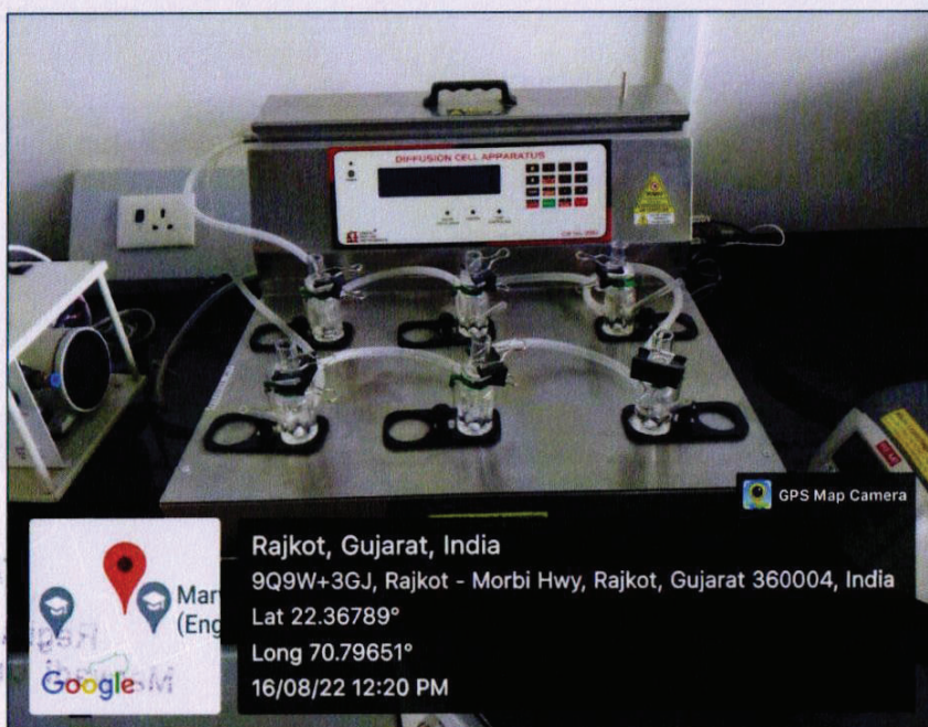
Franz-diffusion cell apparatus
